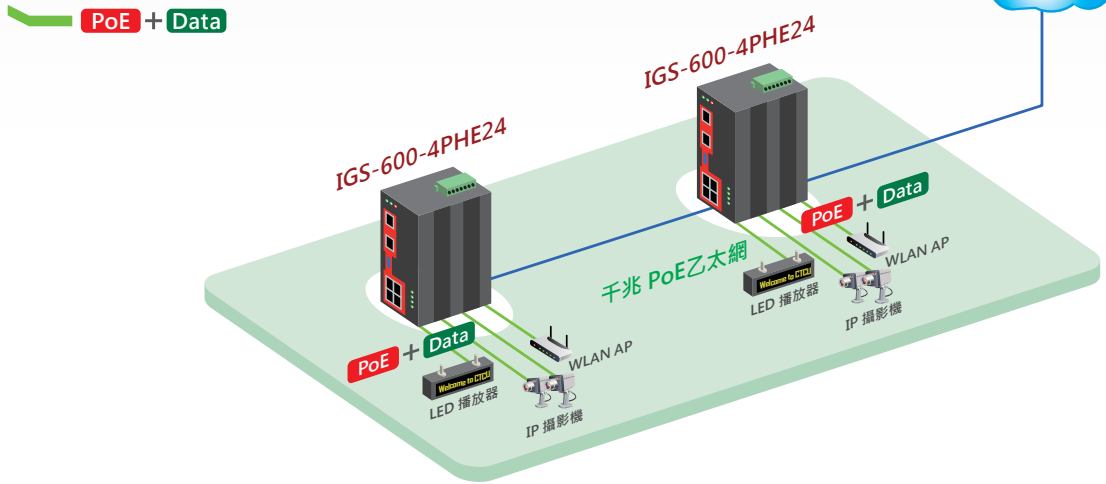
IGS-600-4PH24 PoE 乙太網交換機傳輸連線圖
